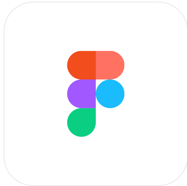
Figma
